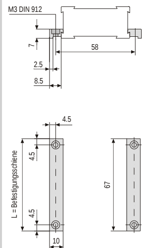
Befestigungssatz B Fastening set B
